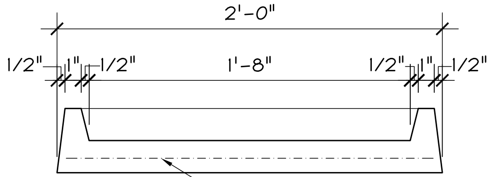
ELEVATION
